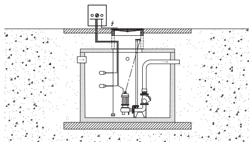
Principe opstelling P1000 serie beton
