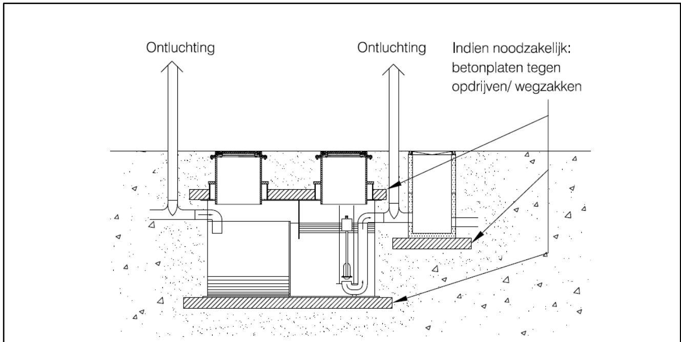
Figuur 1 – Principeopstelling plaatsing KPE.MI 6000 HV/E.
