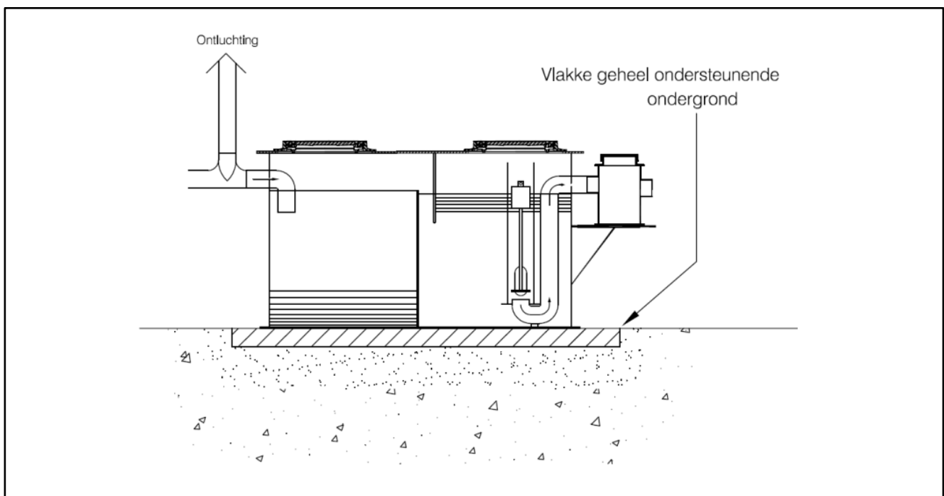
Figuur 2 – Principeopstelling plaatsing KPE.MI 6000 BG.
